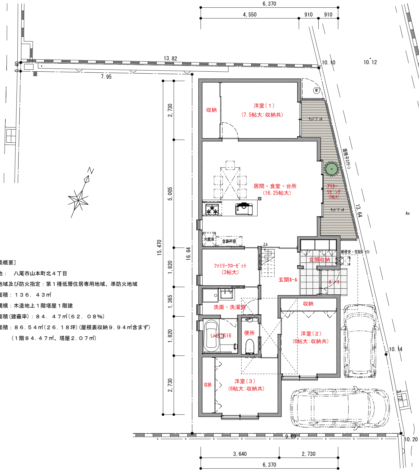
配置図兼1階平面図
