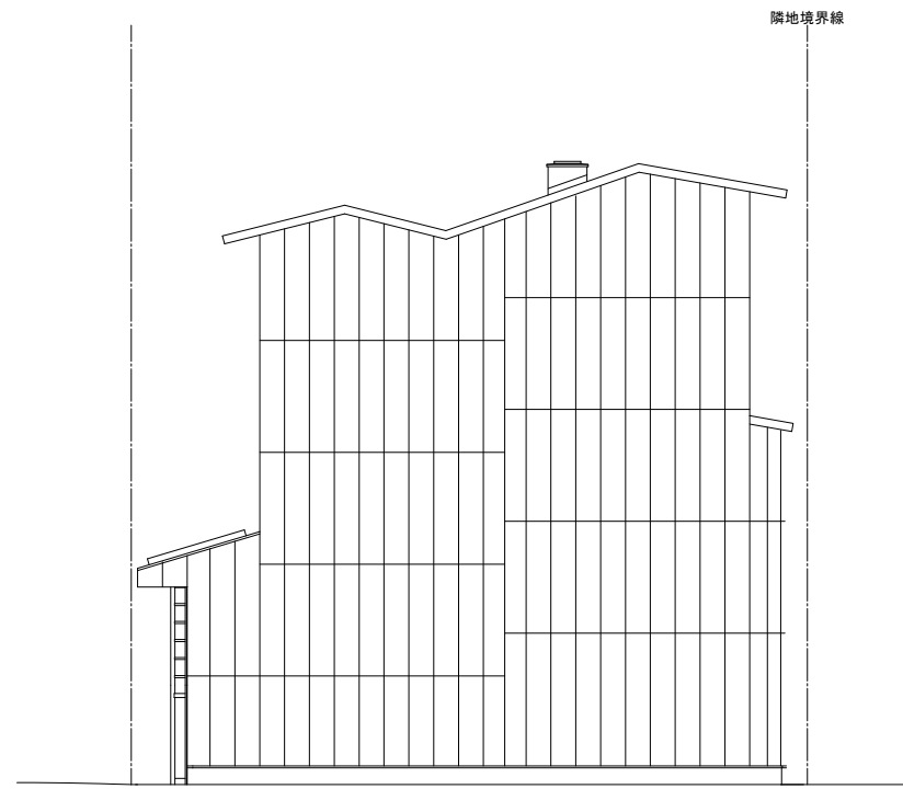
西立面图
