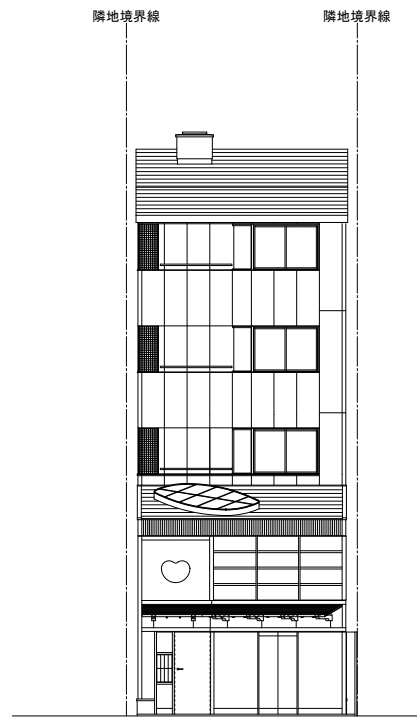
北立面图
