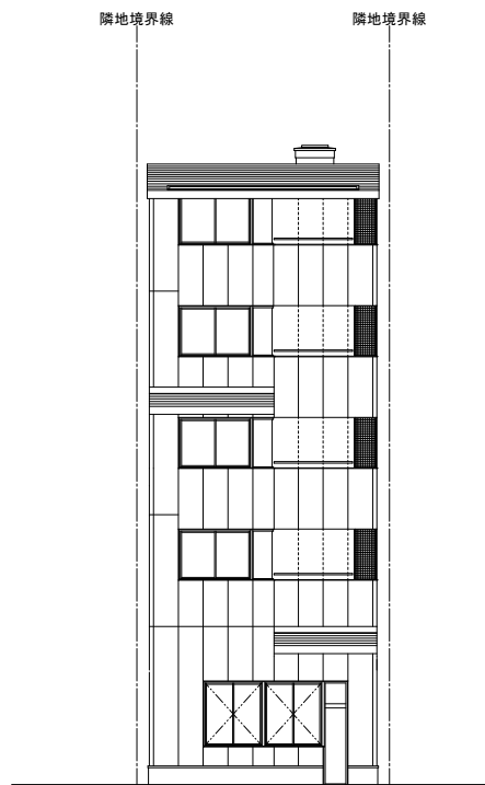
南立面图
