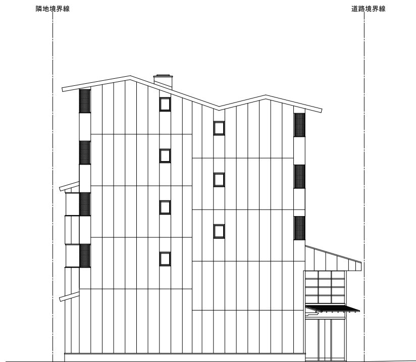
東立面图
