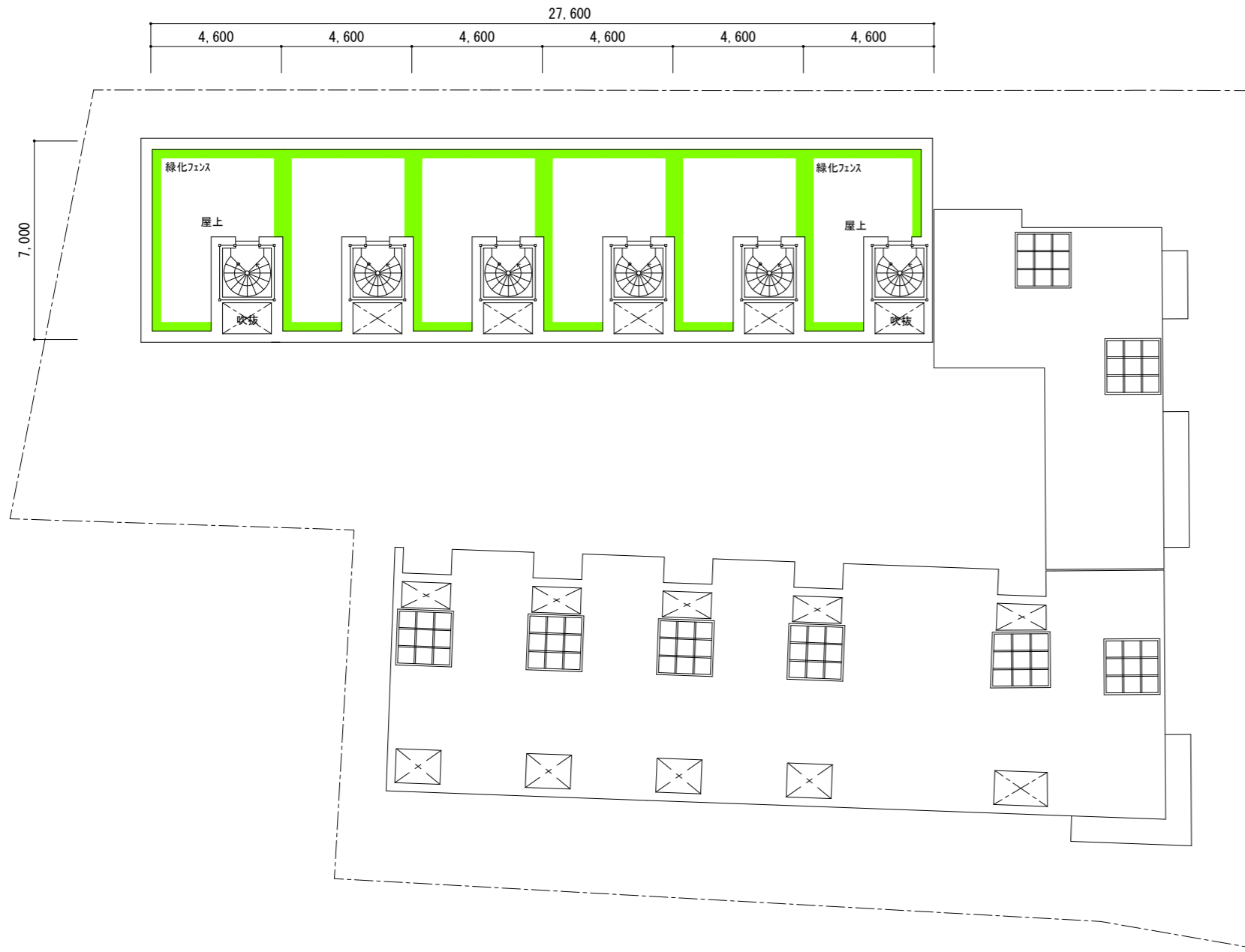
A7' ロックP H 1 階平面図 1/200 —レヴェル5—
