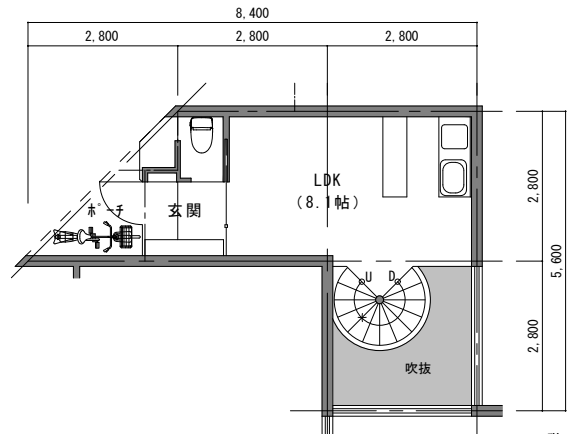
1 階平面図
