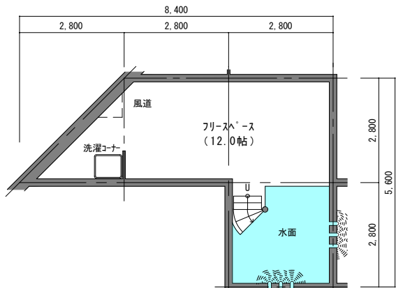
地階平面図
