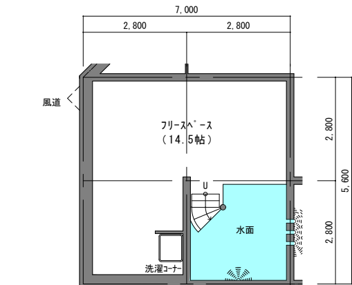
地階平面図
